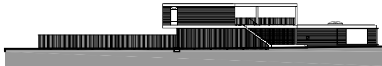
West gevel
