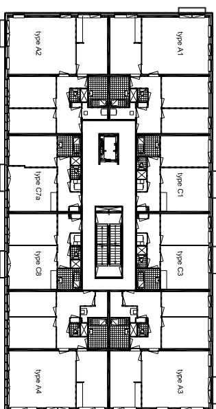
plattegrond blok 1 3e verdieping
