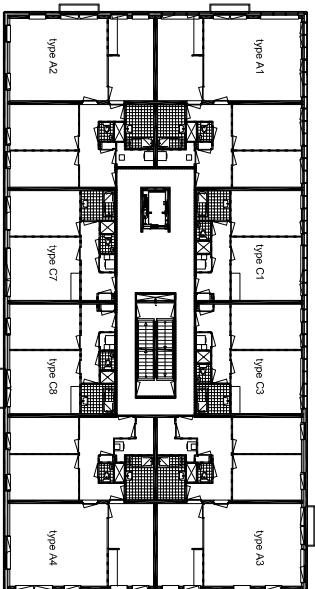
plattegrond blok 1 2e verdieping
