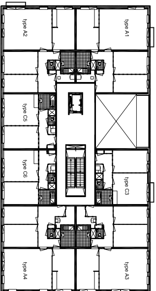
plattegrond blok 1 1e verdieping
