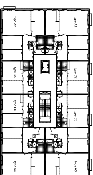
plattegrond blok 1 7e verdieping
