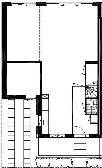
woningtype H begane grond
