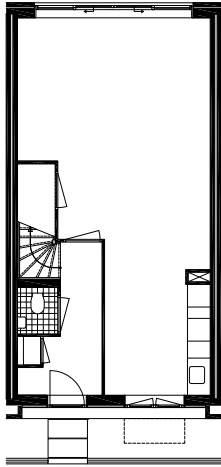
woningtype E begane grond
