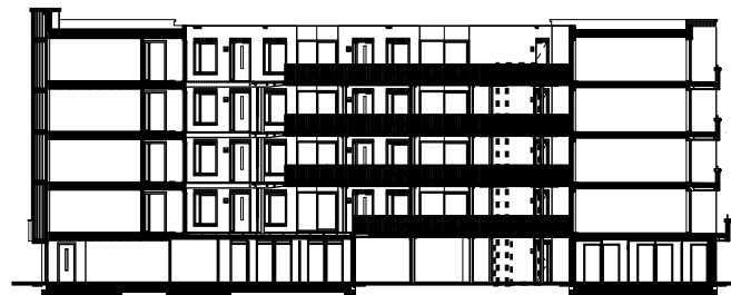
Doorsnede D-D
