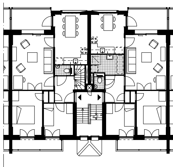
1e verdieping
