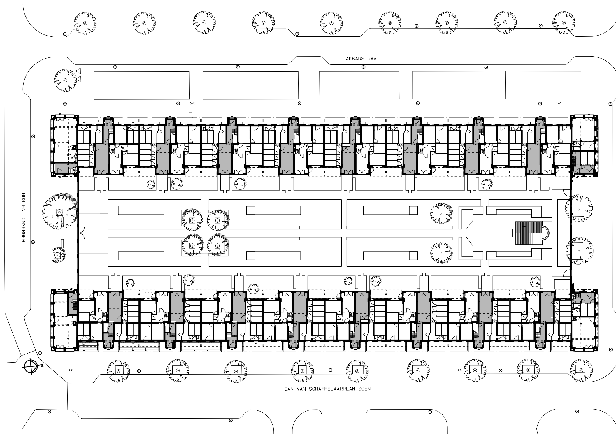
situatie blok
