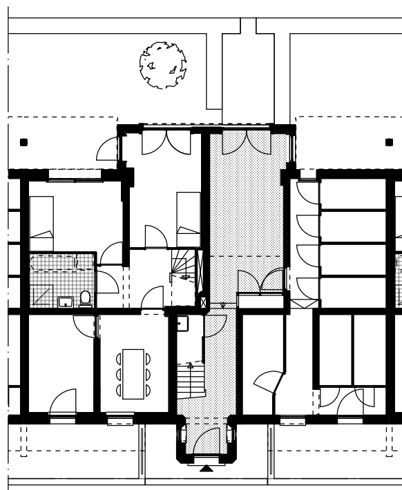
begane grond
