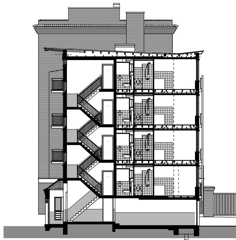
doorsnede over bestaand portiek, nieuw toilet, badkamer en keuken
