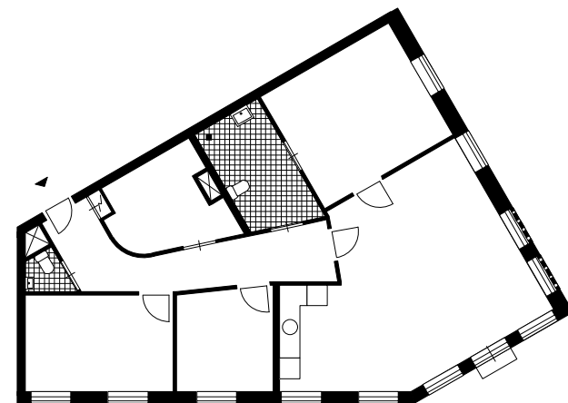
Woningtype E (rowo) (1e, 2e, 3e, 4e)- GBO: 81,6m 2
