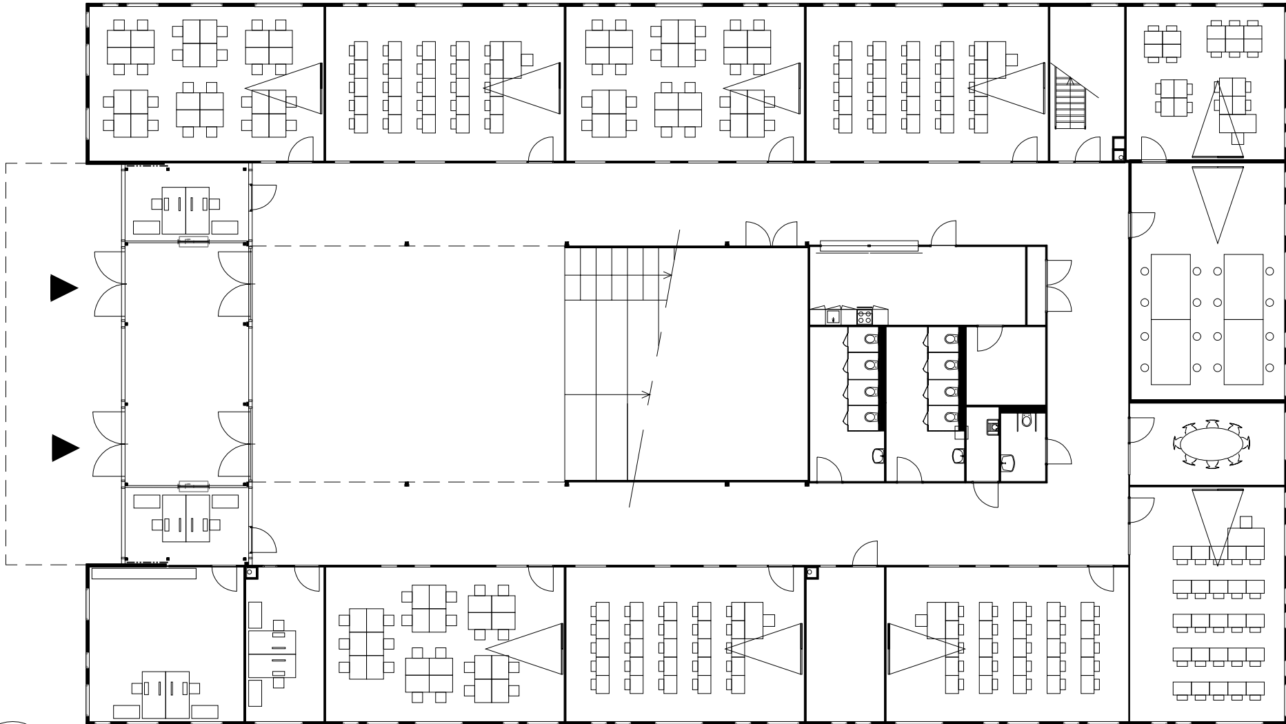
Begane grond
