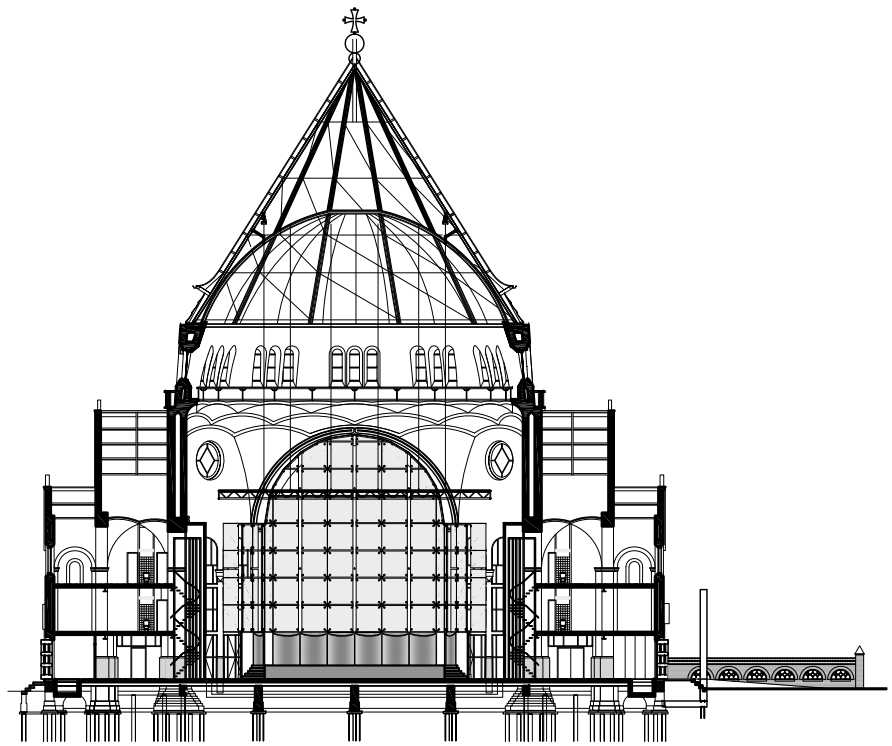
Dwarsdoorsnede
