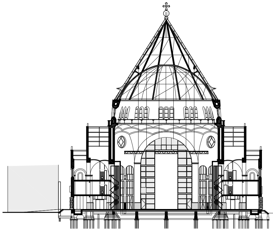
Dwarsdoorsnede
