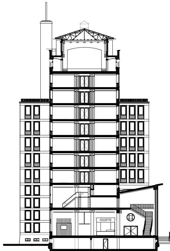
DOORSNEDE KOHNSTAMMHUIS
