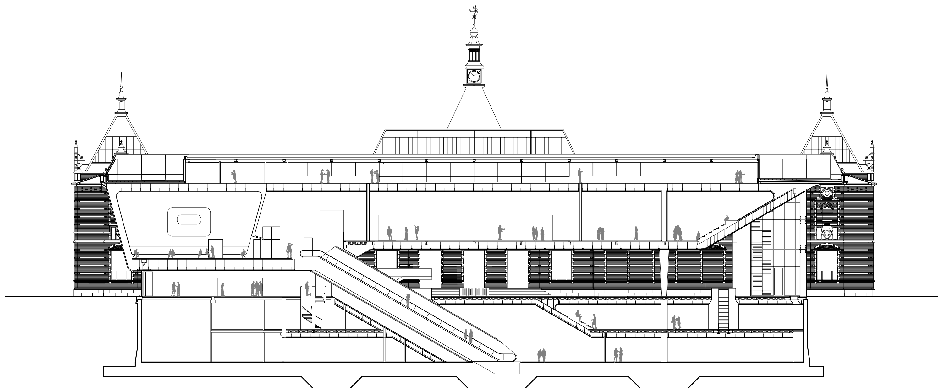
Longitudinal section
