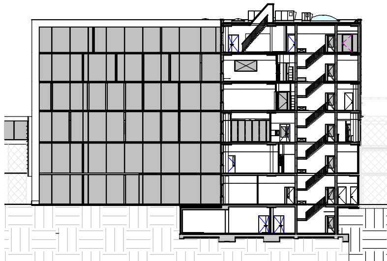
doorsnede D-D 1:500
