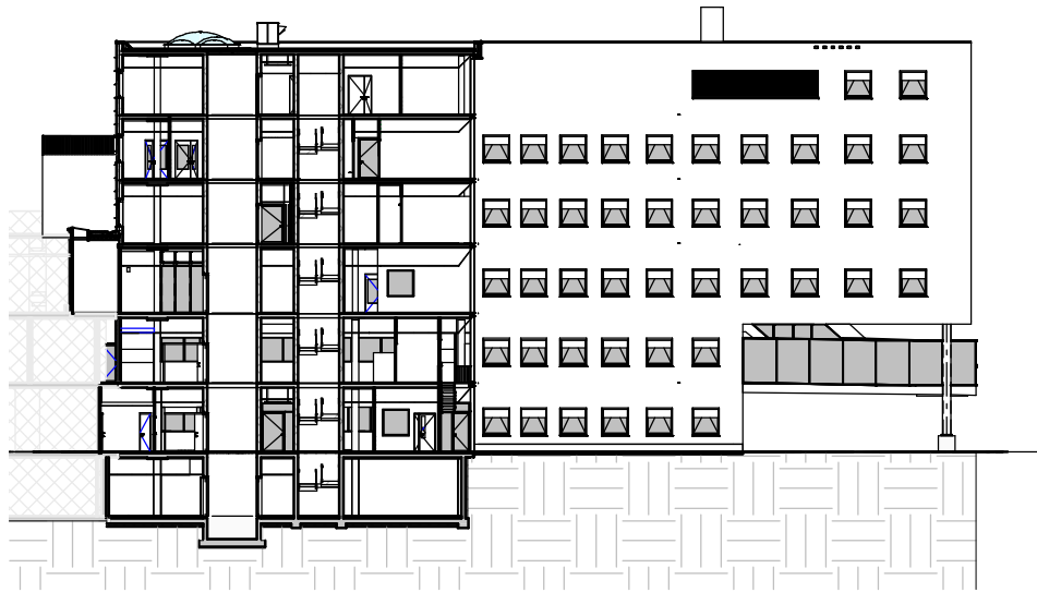
doorsnede C-C 1:500
