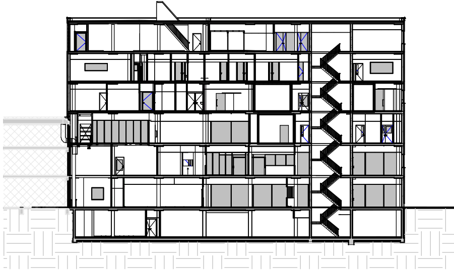
doorsnede A-A 1: 500
