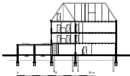
doorsnede linkerzijvleugel 1:500
