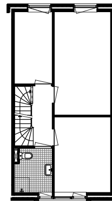
1e verdieping
