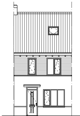
Voorgevel
