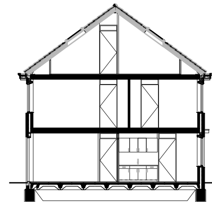
Doorsnede
