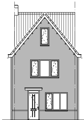
Voorgevel
