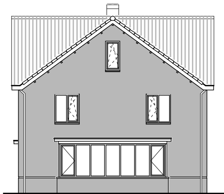
Zijgevel rechts
