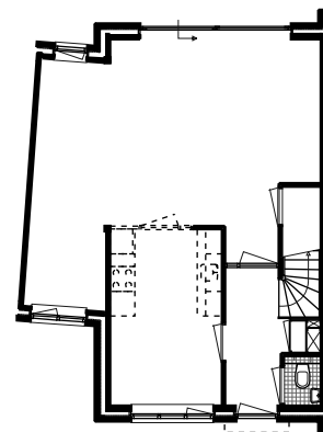
Begane grond
