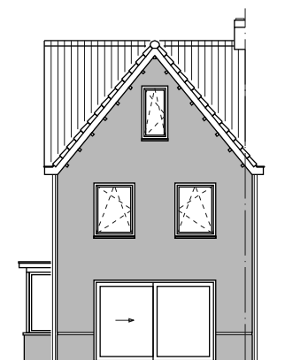
Achtergevel
