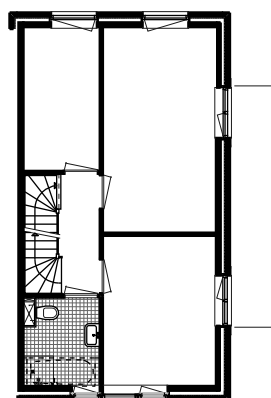
1e verdieping
