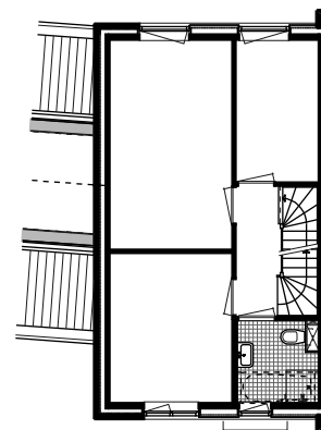
1e verdieping
