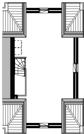
2e verdieping
