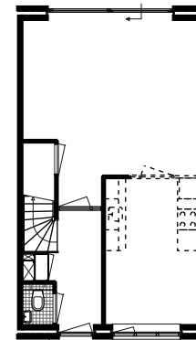
Begane grond
