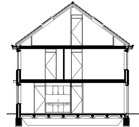
Doorsnede
