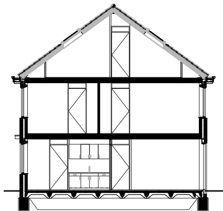
Doorsnede
