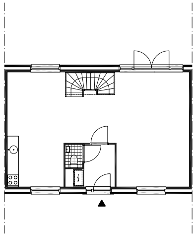
begane grond
