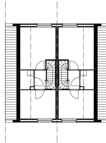
tweede verdieping
