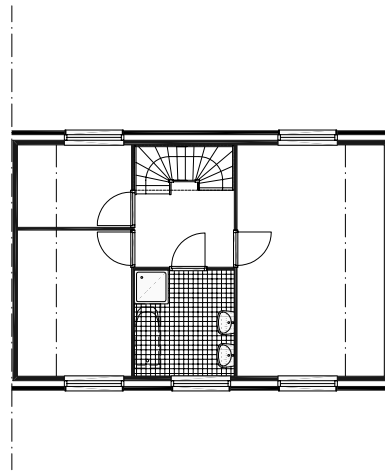
eerste verdieping
