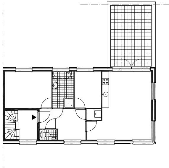
eerste verdieping
