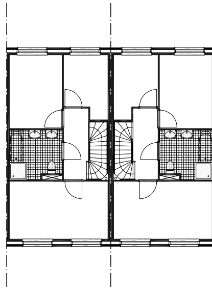
eerste verdieping
