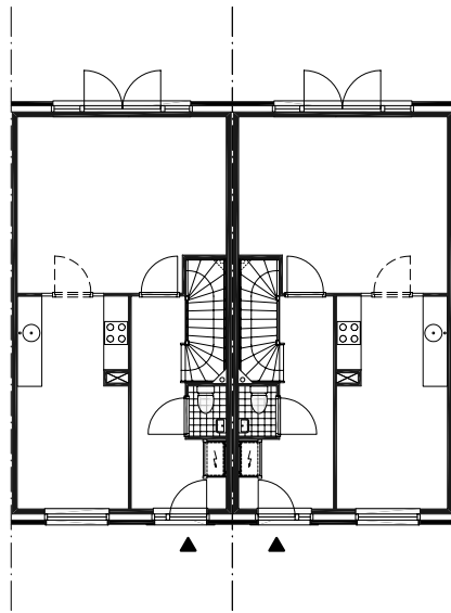
begane grond
