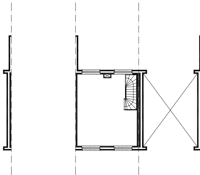
eerste verdieping
