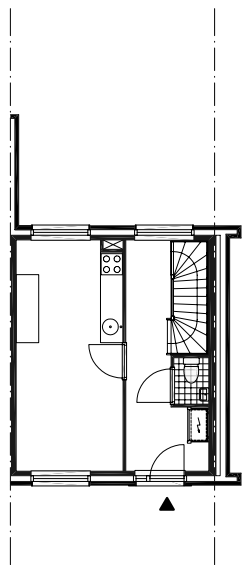
begane grond
