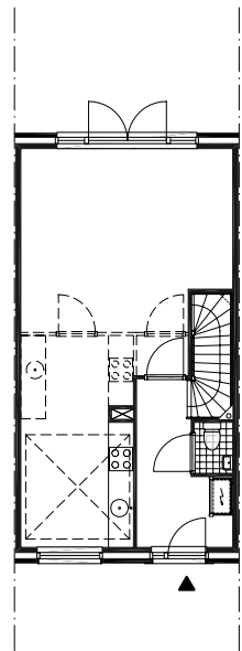
begane grond
