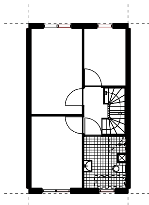
eerste verdieping
