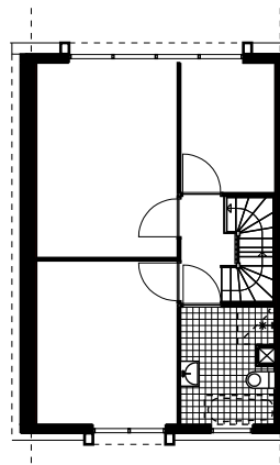
eerste verdieping
