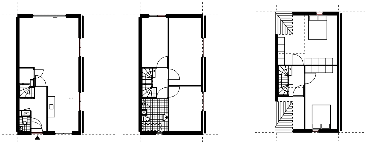
begane grond
