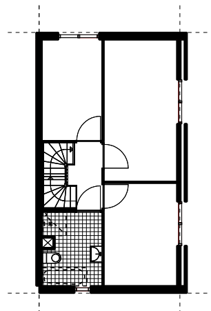
eerste verdieping
