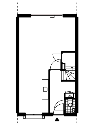
begane grond
