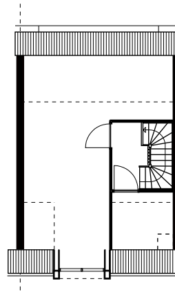
tweede verdieping
