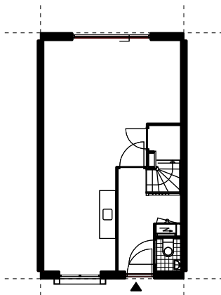
begane grond
