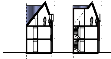
Doorsnede type F1
