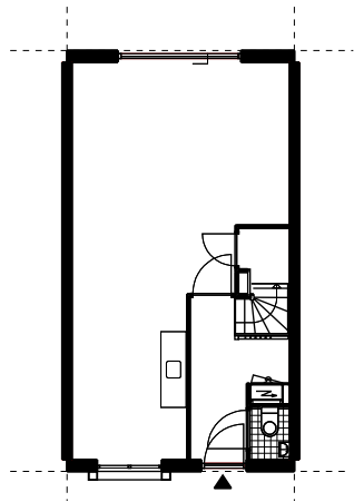
begane grond
