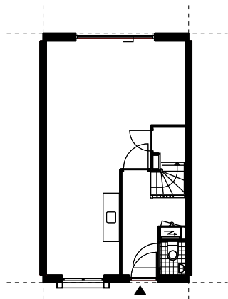
begane grond
