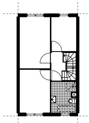
eerste verdieping
