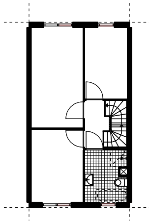
eerste verdieping
