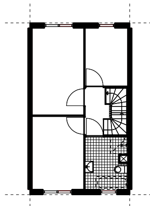
eerste verdieping
