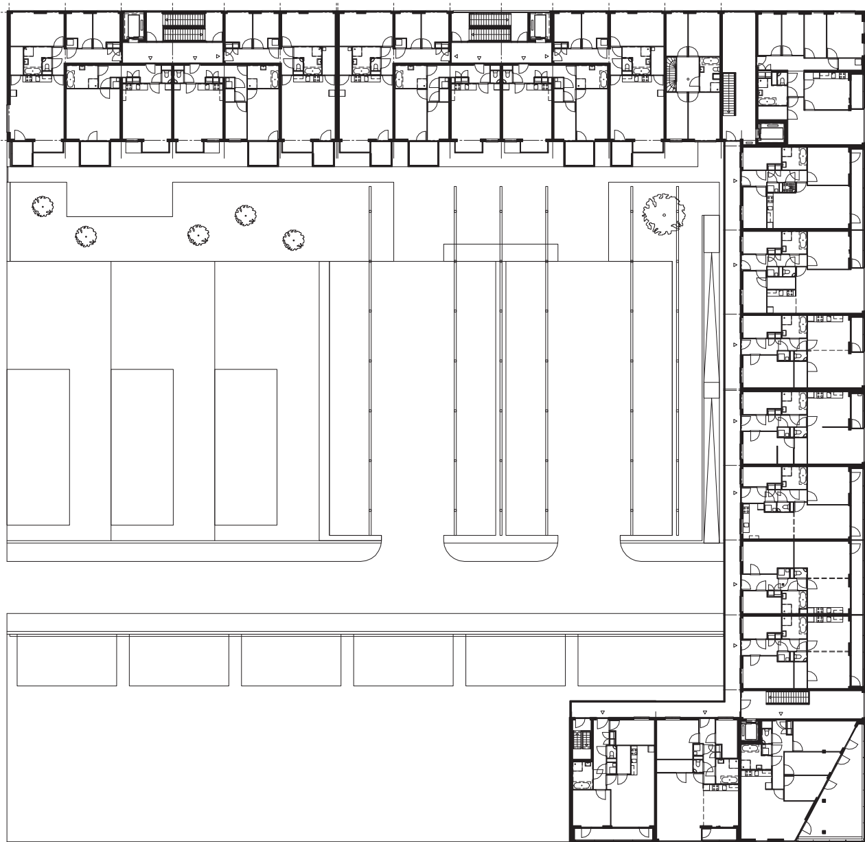
Plattegrond 3e verdieping
