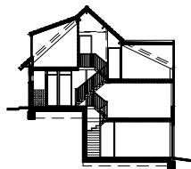
doorsnede 1:500
