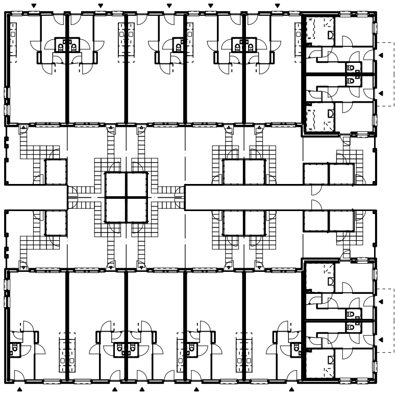
BEGANE GROND schaal 1:500
