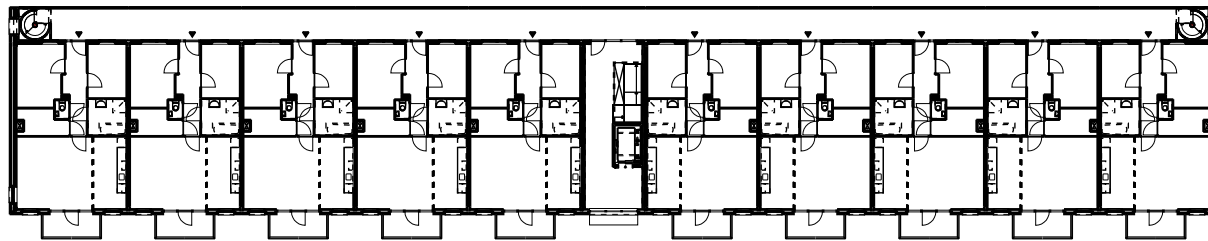
2e & 3e VERDIEPING schaal 1:500
