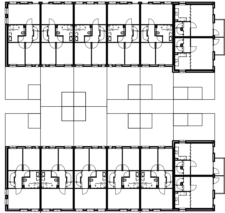
1E VERDIEPING schaal 1:500
