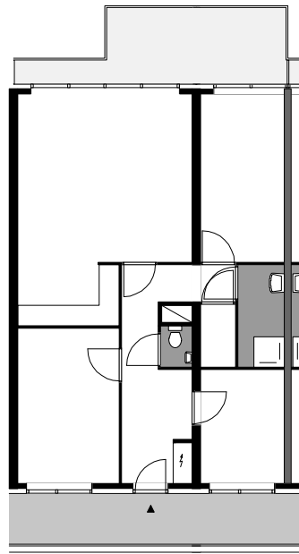
type E4 1:100
