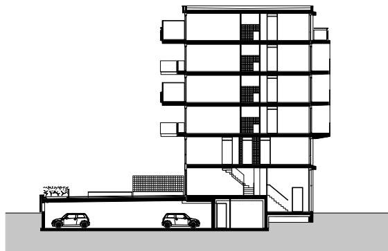
DOORSNEDE
