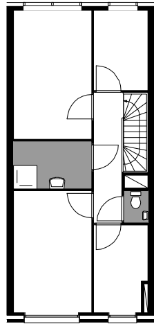
type D1 1:200
