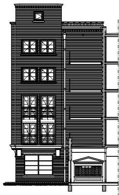
voorgevel 1
