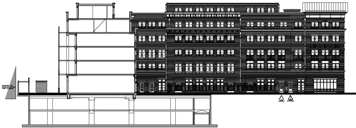
doorsnede D
