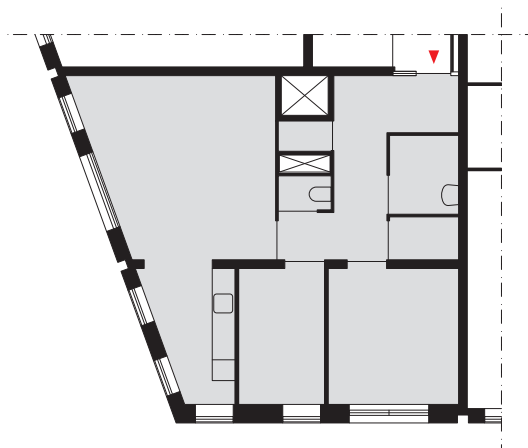
WONINGTYPE H
