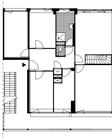
TYPE D MAISONETTE VERDIEPING 1:200 NIVO 0
