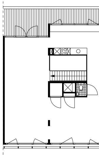
TYPE E TOP MAISONETTE VERDIEPING 1:200 NIVO 5
