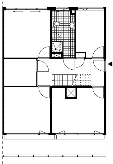
TYPE E TOP MAISONETTE 1:200 NIVO 4
