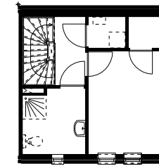
woningtype C 2e verdieping
