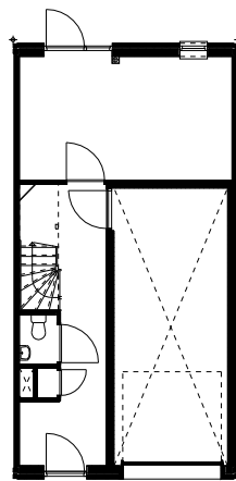
woningtype G begane grond
