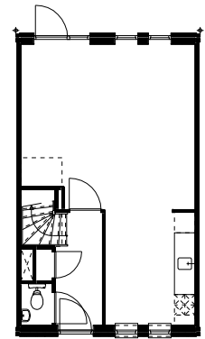
woningtype E begane grond
