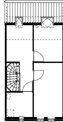
woningtype F 2e verdieping
