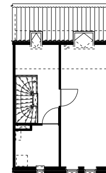
woningtype H 2e verdieping
