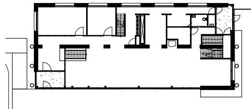
begane grond
