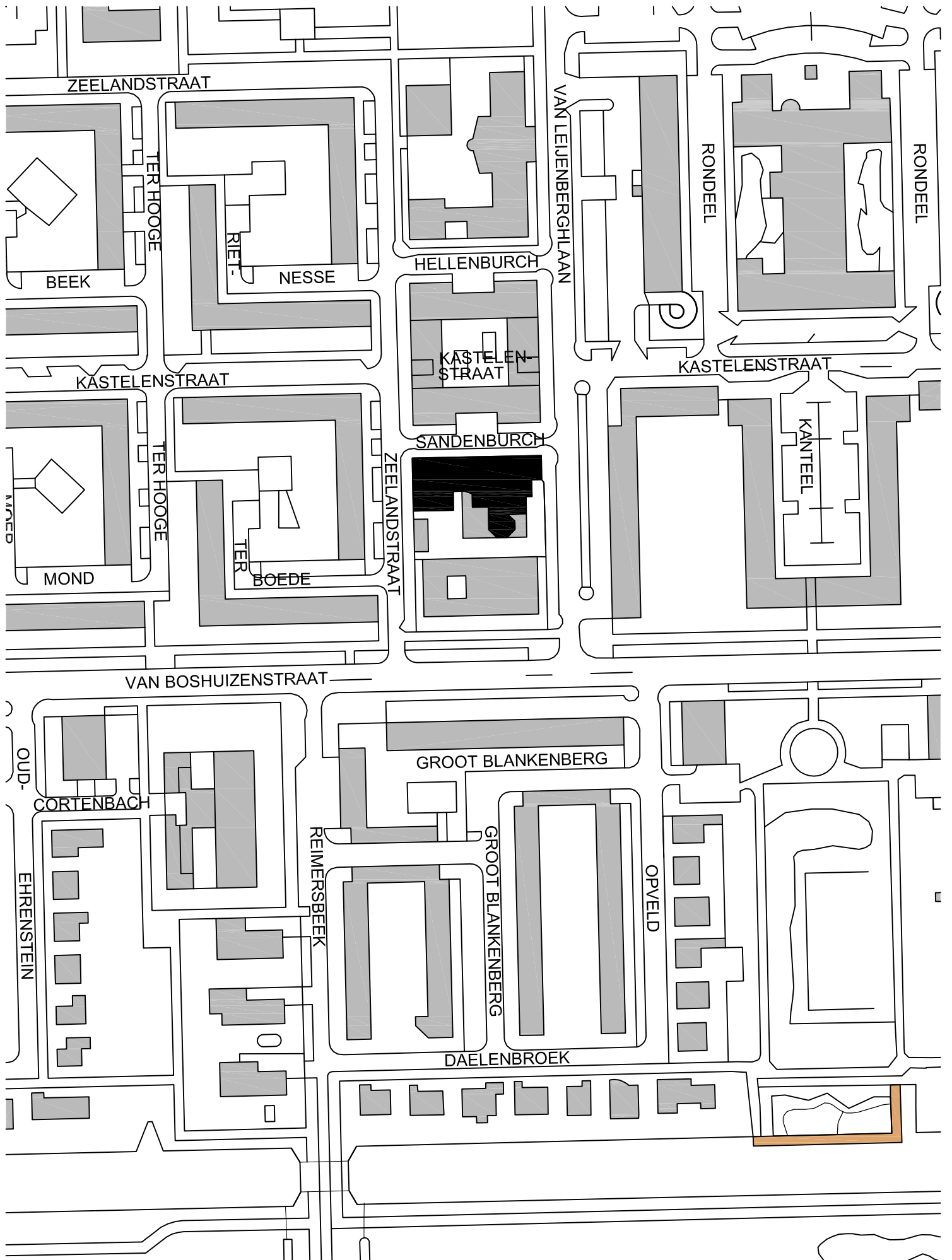
Buitenveldertse Montessorischool situatietekening schaal 1:2000
