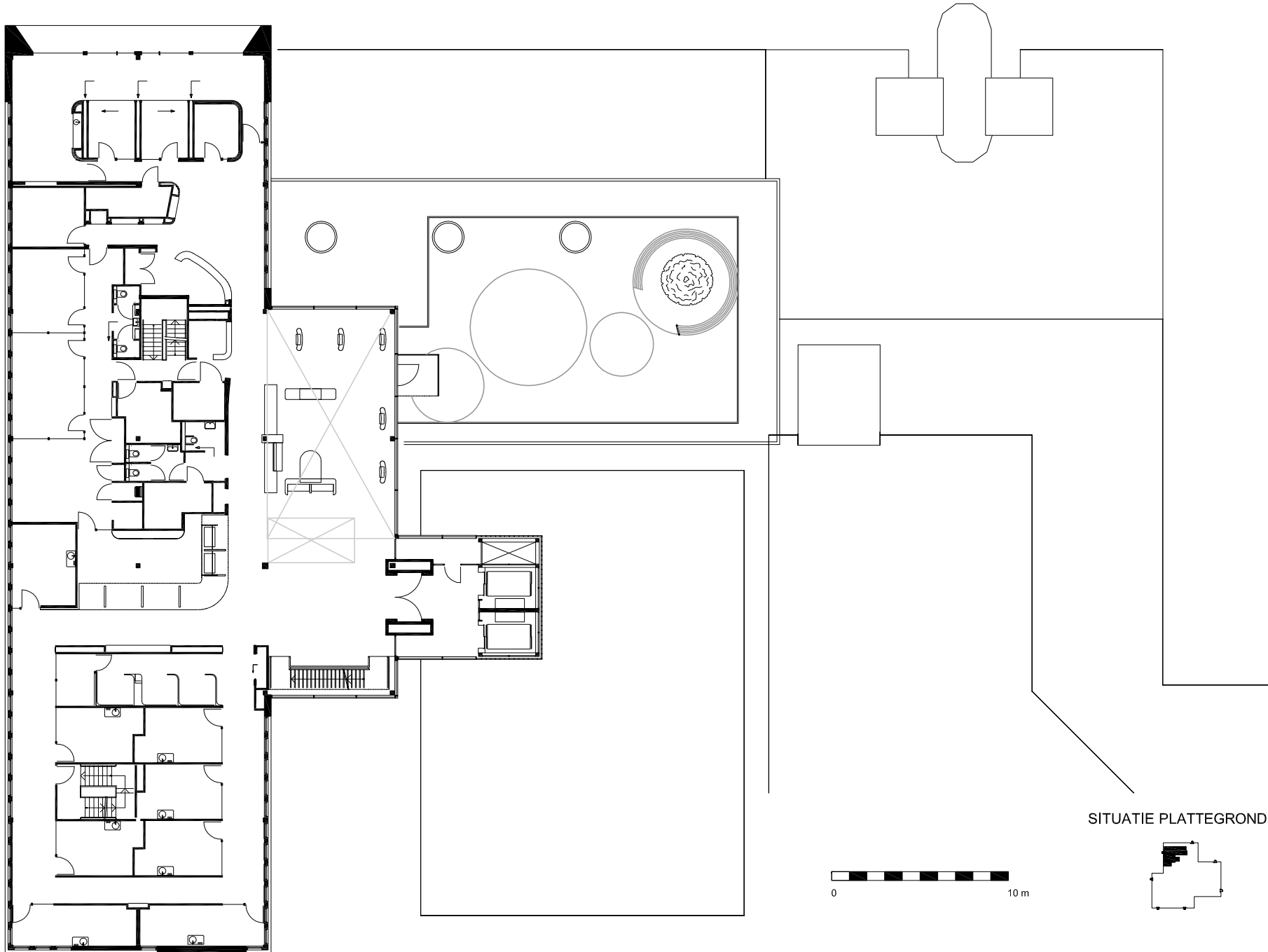
PLATTEGROND 3E BOUWLAAG NIEUWBOUW (6e VERDIEPING)
