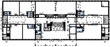
BEGANE GROND
