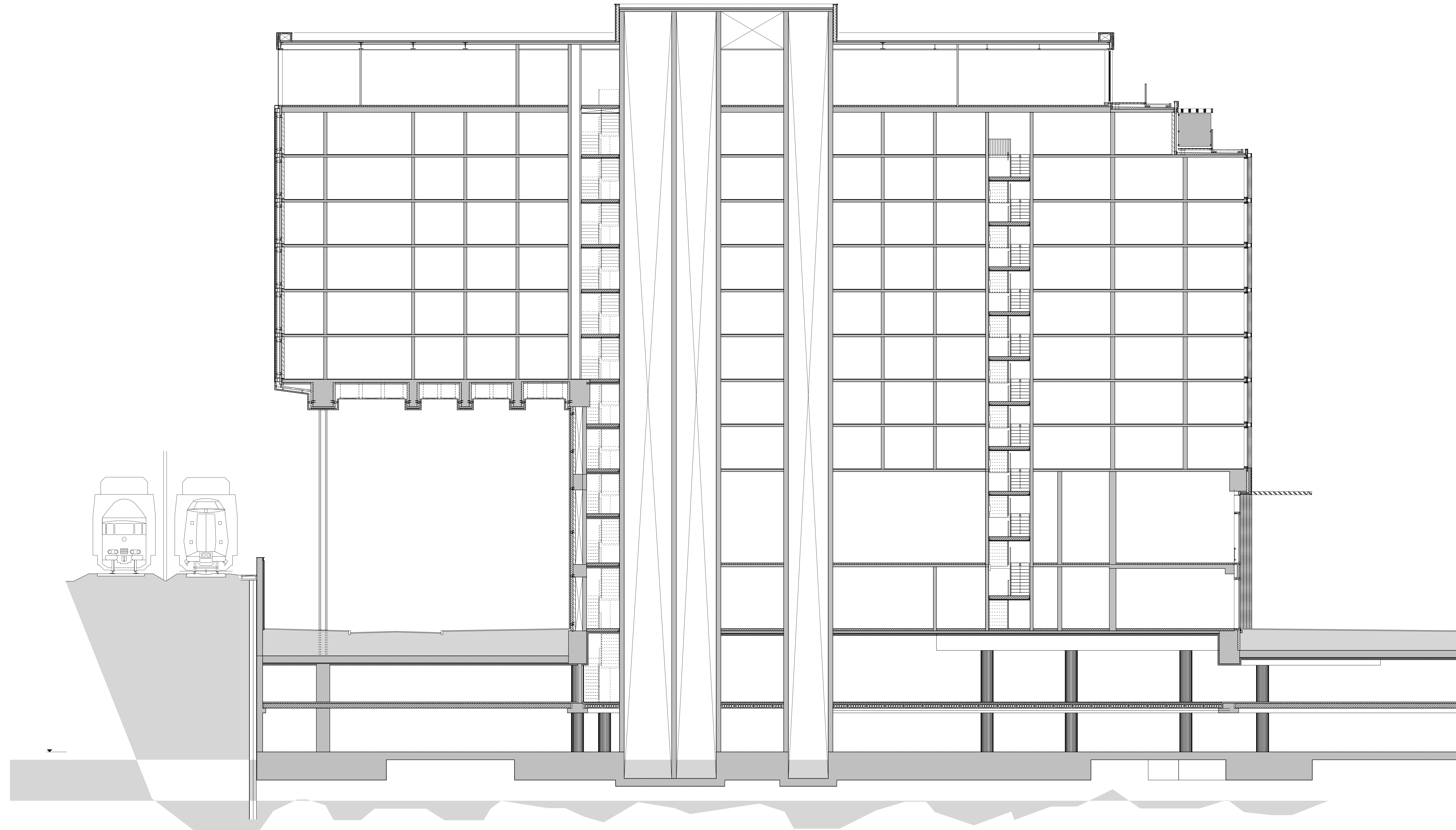
0 5 10 DOORSNEDE
