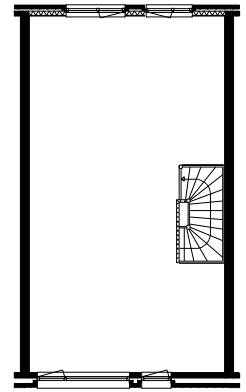
540-3-sh 2e verdieping
