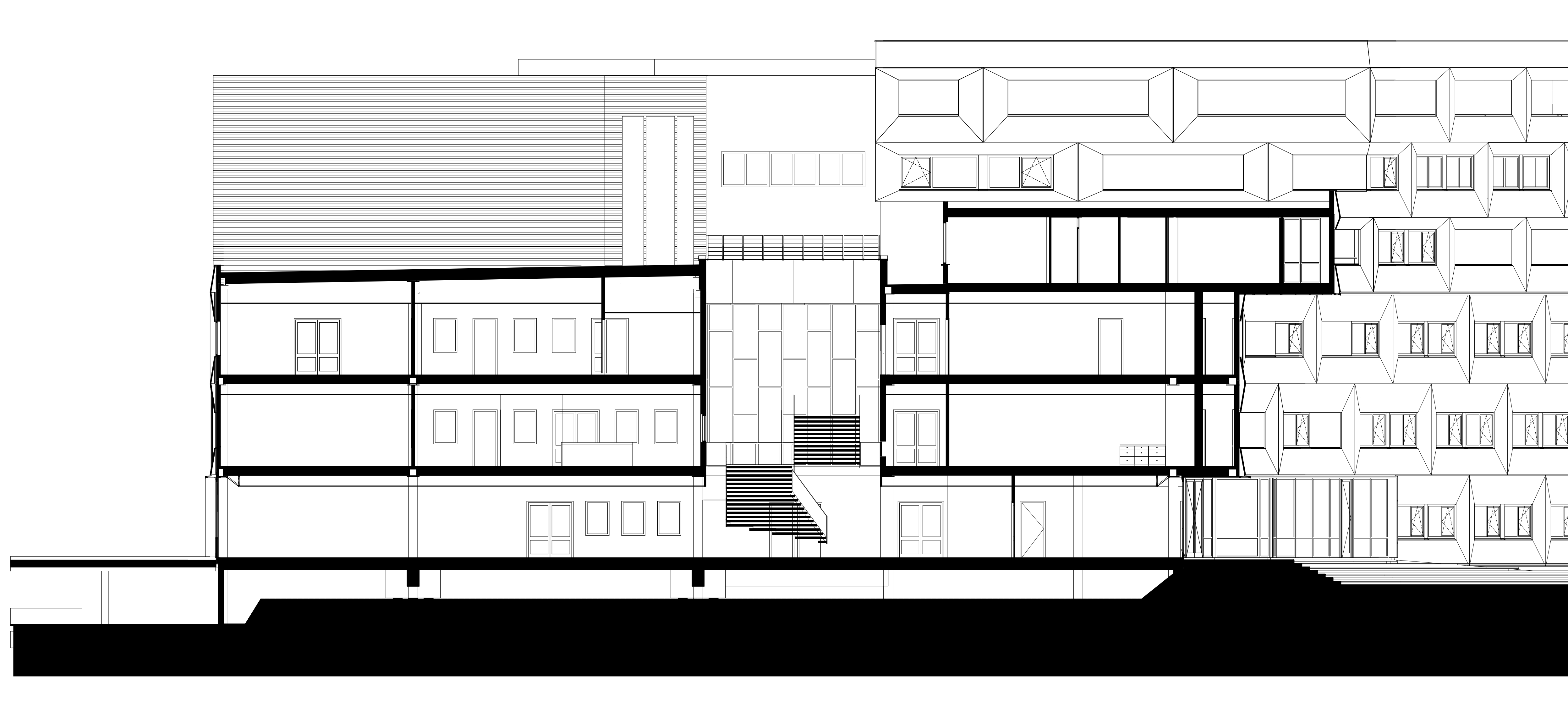
Doorsnede C-C
