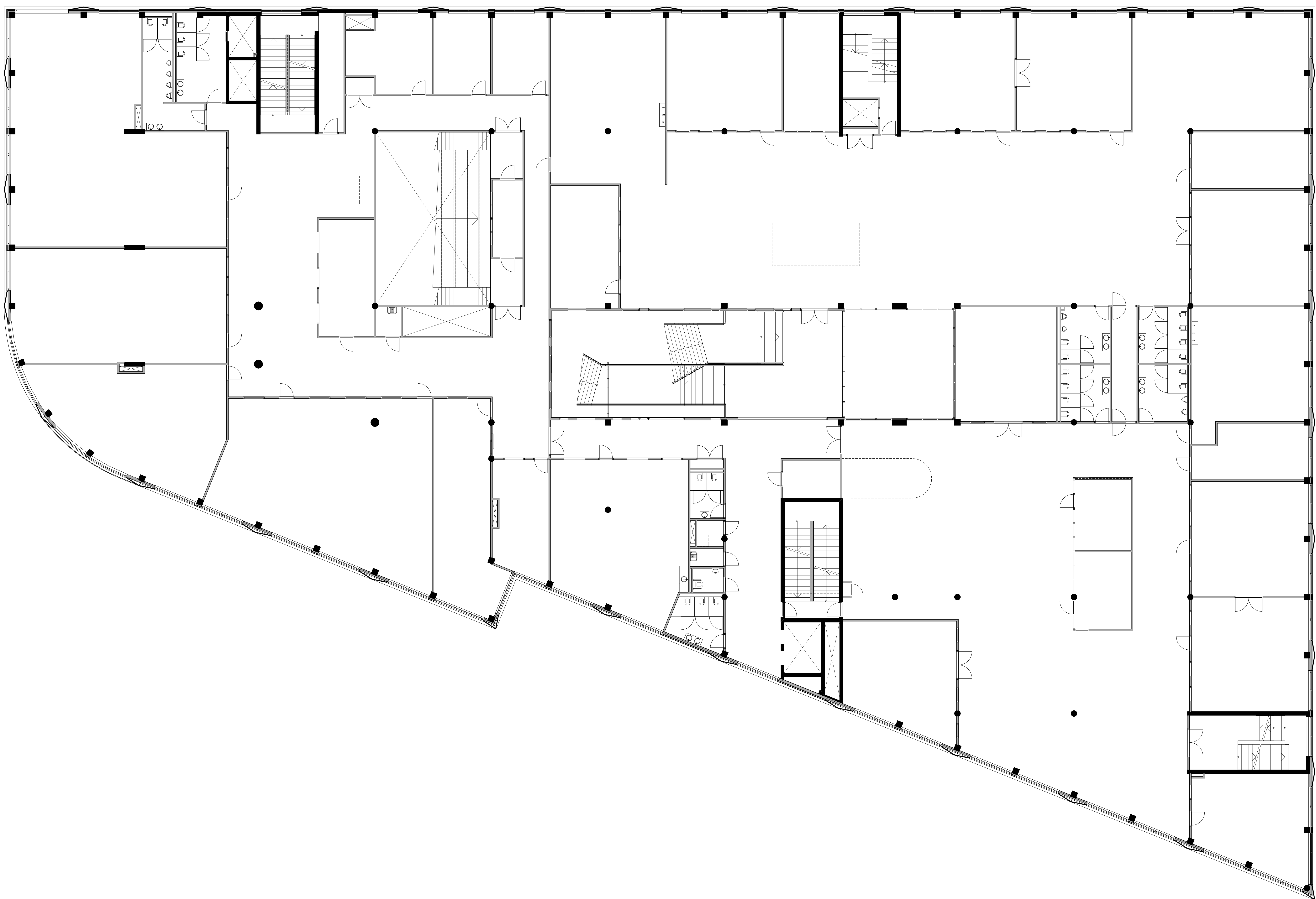
Plattegrond 1e Verdieping
