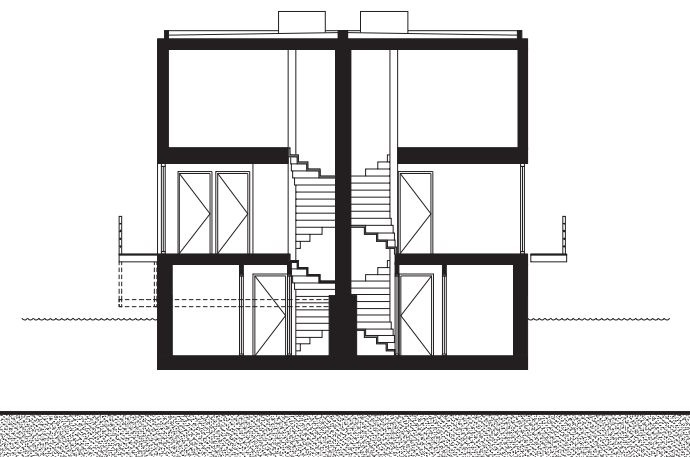
doorsnede B
