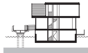
doorsnede B
