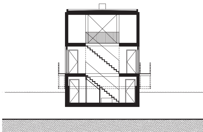
doorsnede B
