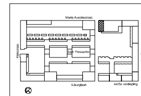
Plattegrond bouwnummer 178 Type E21a
