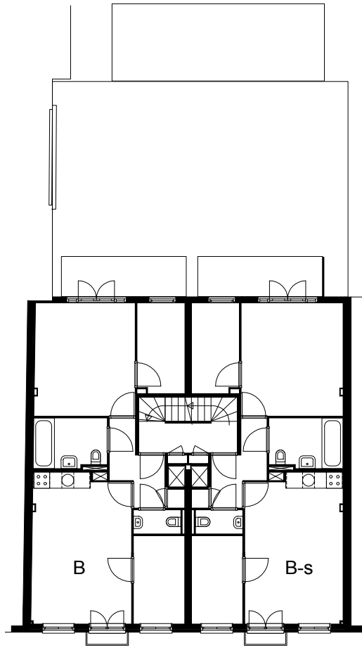
3e verdieping
