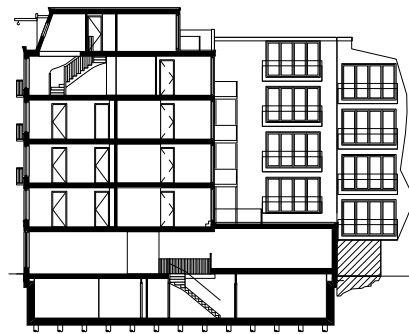
langsdoorsnede
