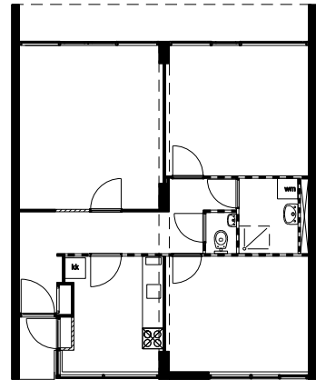
Begane grond
