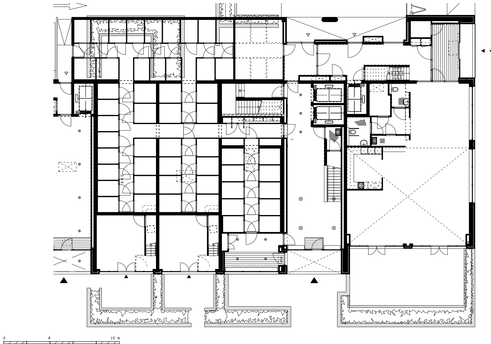
overzicht blok B3, laag 00, entree en zorgsteunpunt
