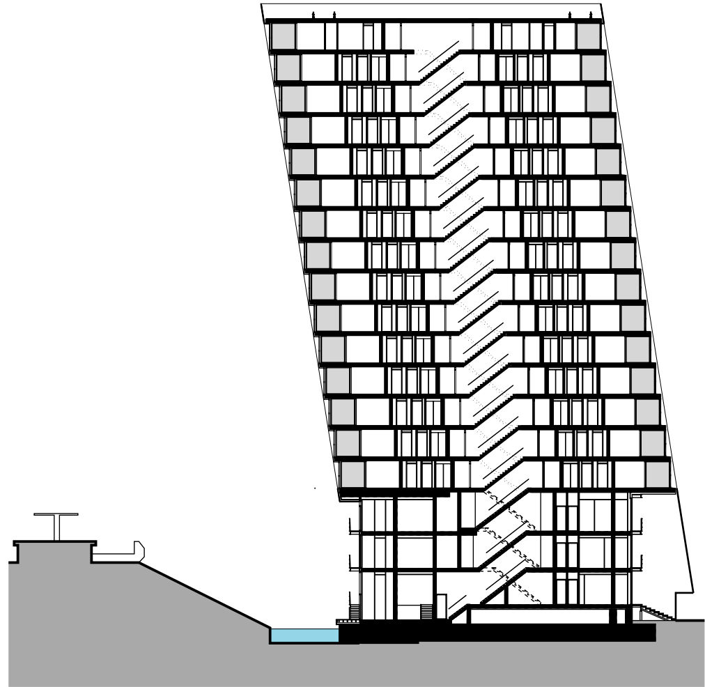
DOORSNEDE schaal 1:500
