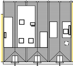
DAKOVERZICHT
