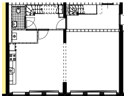
3e VERDIEPING WONINGTYPE A5
