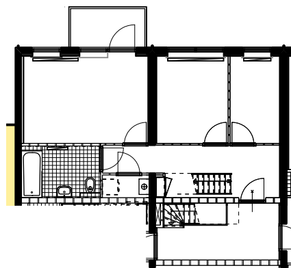
3e VERDIEPING WONINGTYPE A6
