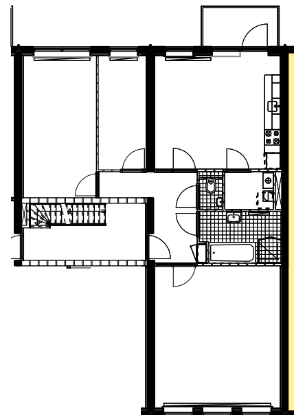
2e VERDIEPING WONINGTYPE A4
