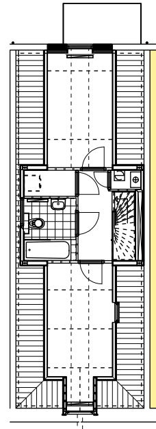
4e VERDIEPING WONINGTYPE A7
