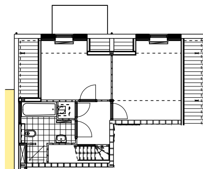
4e VERDIEPING WONINGTYPE A5
