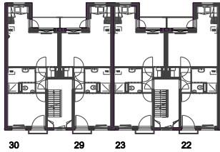
1ste VERDIEPING
