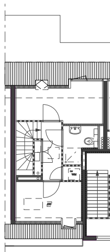
4e verdieping
