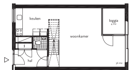
begane grond type E1 gbo: 86.8 m²
