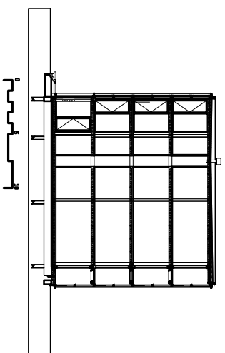
doorsnede 1
