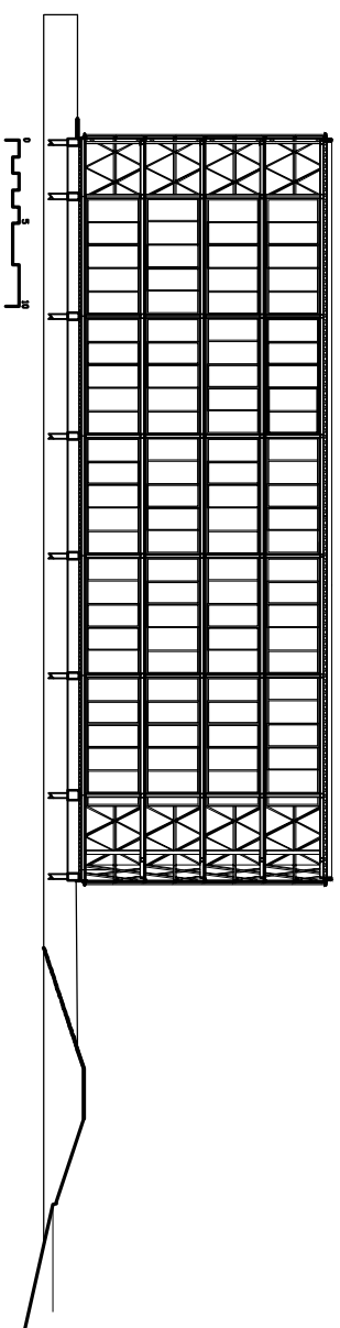
doorsnede B
