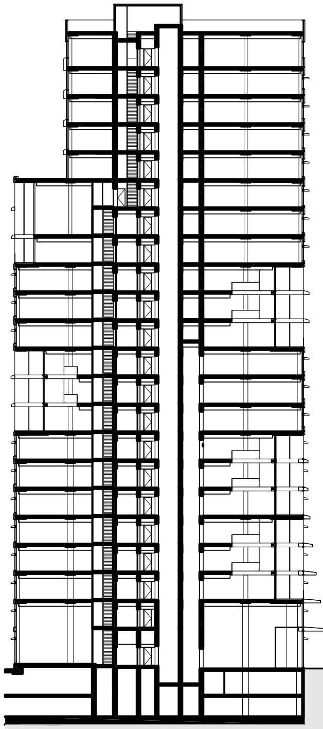
Langsdoorsnede
