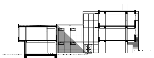
DOORSNEDE A-A
