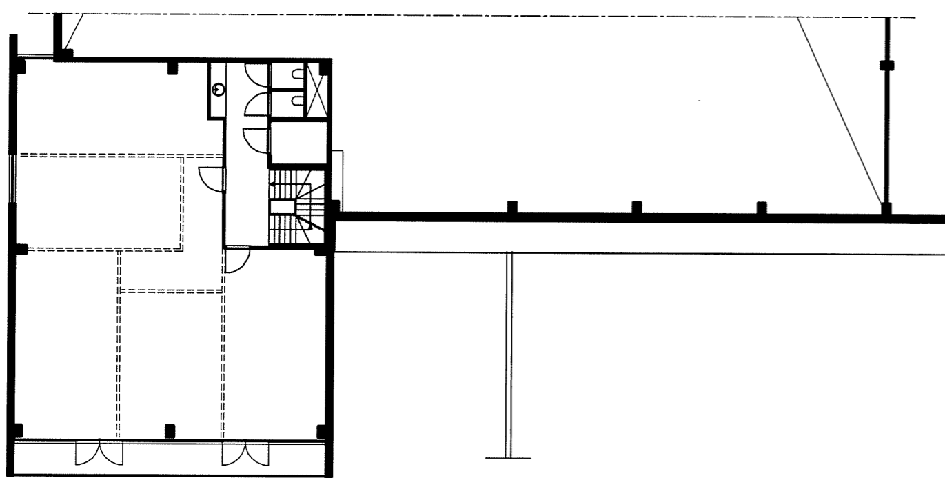
1e Verdieping
