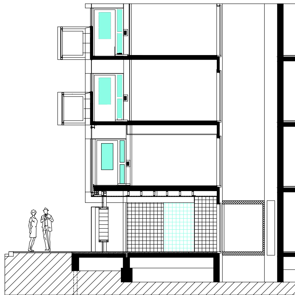
DOORSNEDE AA
