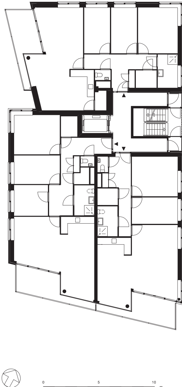
2e t/m 8e verdieping - blok 10 en 11
