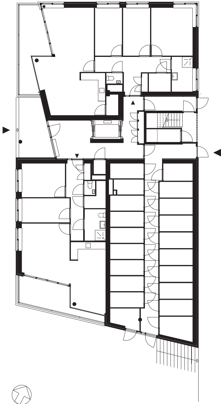
begane grond - blok 10
