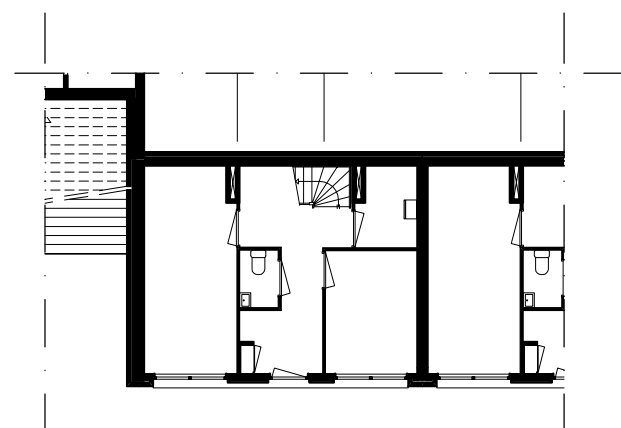
Eengezinswoning laag 1
