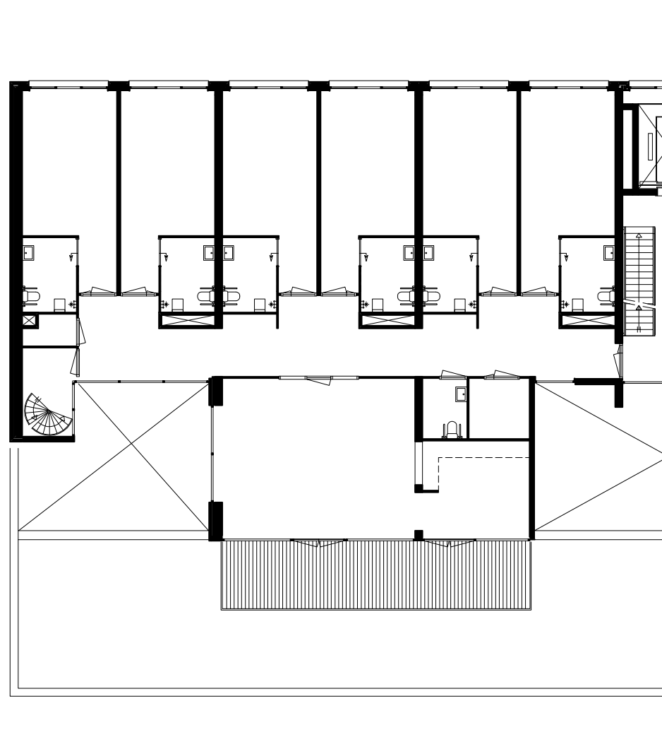
Groepswoning
