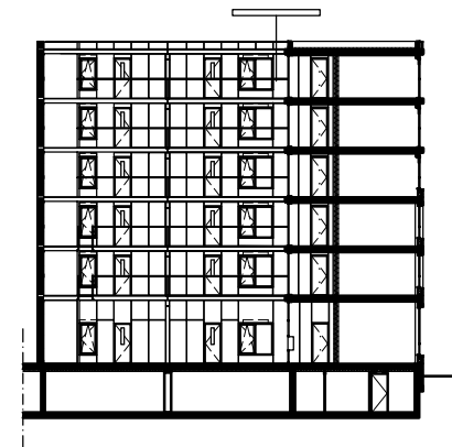
Langsdoorsnede G3
