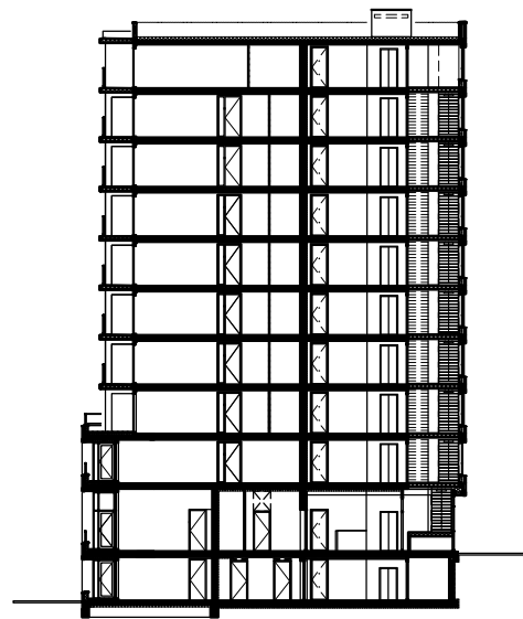
Dwarsdoorsnede G1
