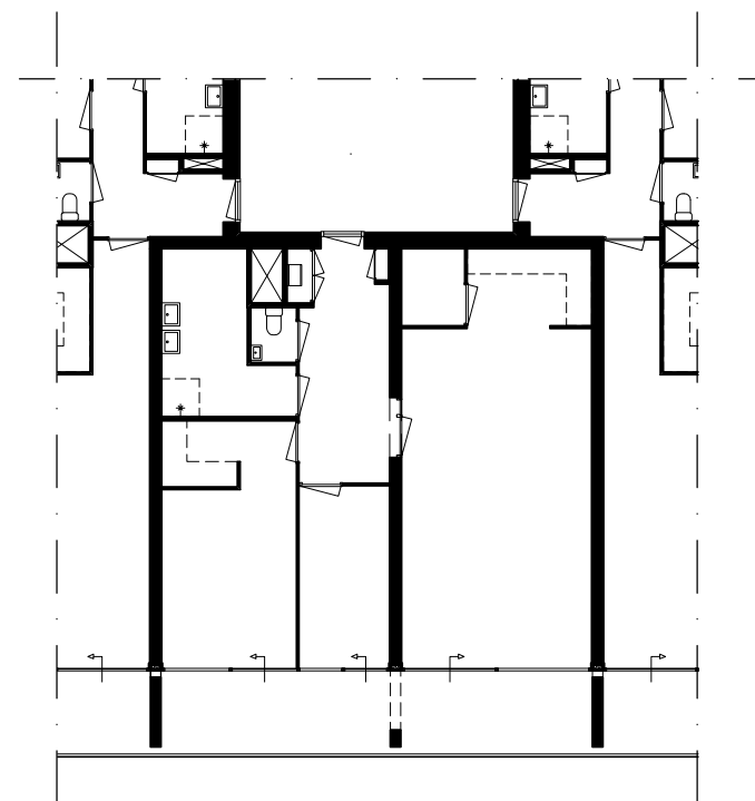
Koop appartement
