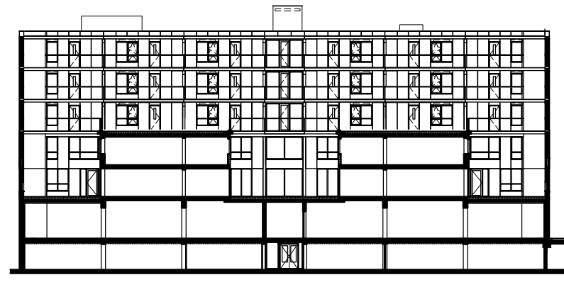
Langsdoorsnede G2
