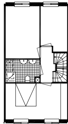
1e verdieping
