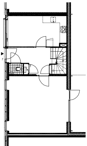
begane grond
