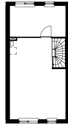
2e verdieping
