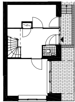
Begane grond
