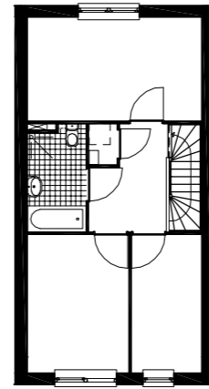
2e verdieping
