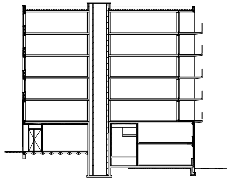
Doorsnede type 2A en 2C
