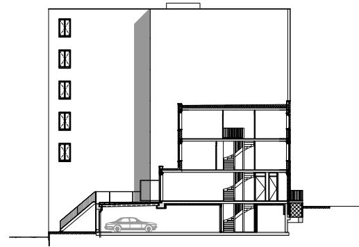
Doorsnede type 1a
